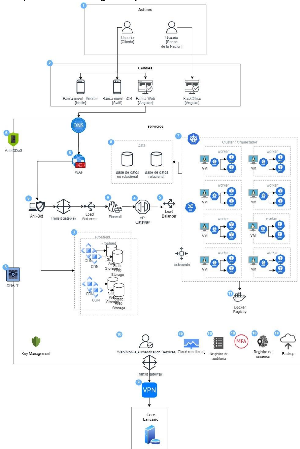
Ilustración 29: Arquitectura Tecnológica para la Banca Móvil y Banca por Internet del Banco de la Nación (diagrama referencial)
